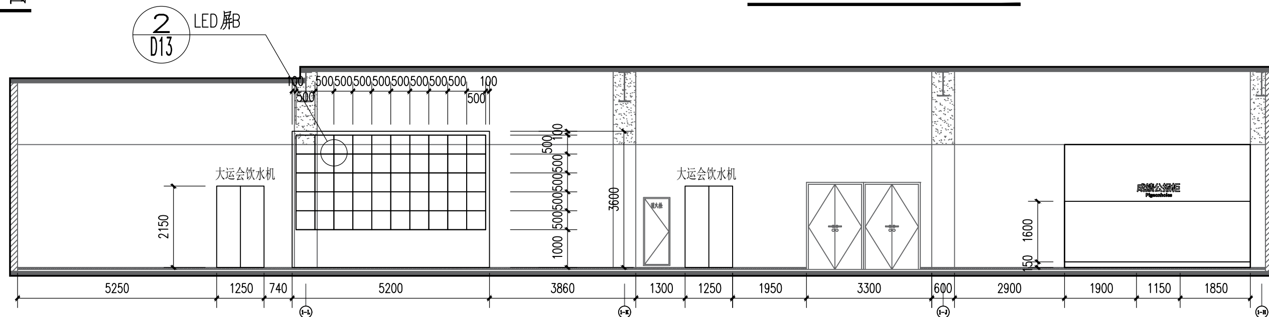
媒体工作间 B立面图 1:100
