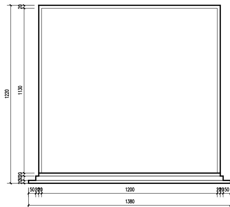
隔断 前视图 1:15
