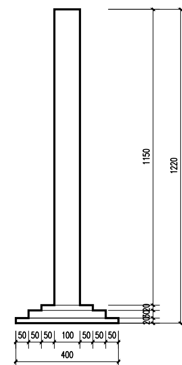
隔断 侧视图 1:15
