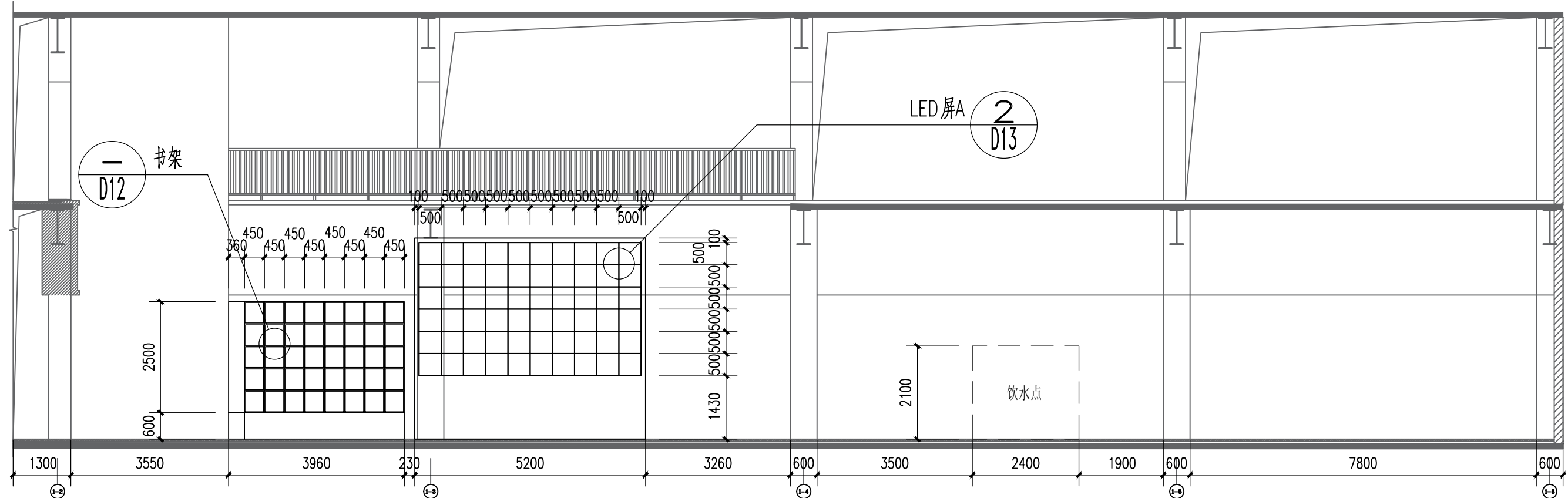
媒体工作间 A立面图 1:100
