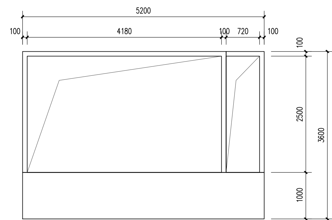
LED屏B 背视图 1:50
