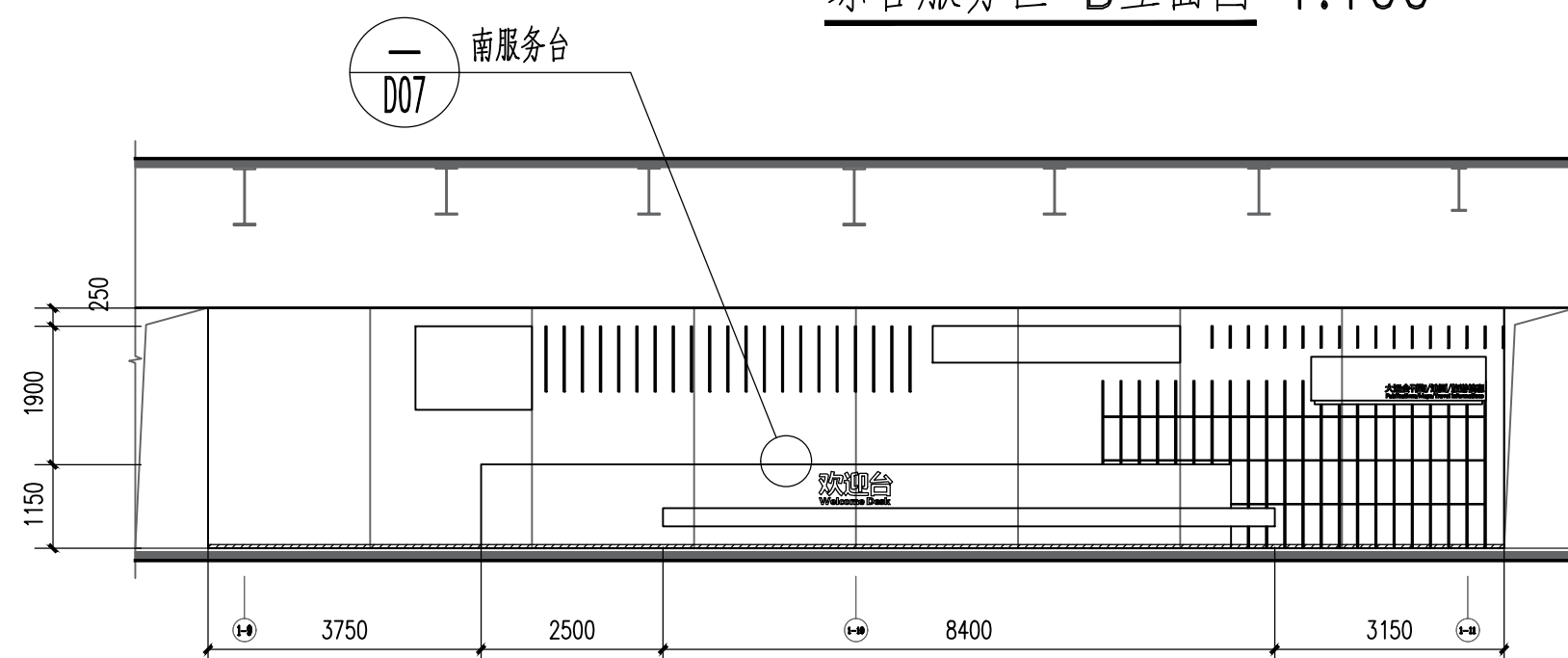
综合服务区 C立面图 1:100
