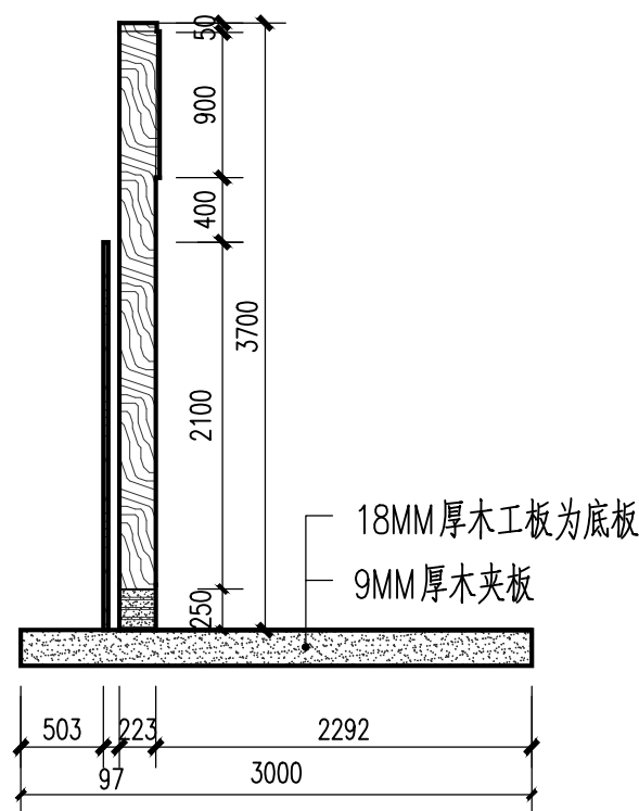
川剧表演舞台侧视图 1:50
