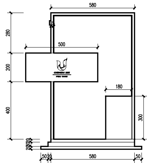
A花箱 前视图 1:15
