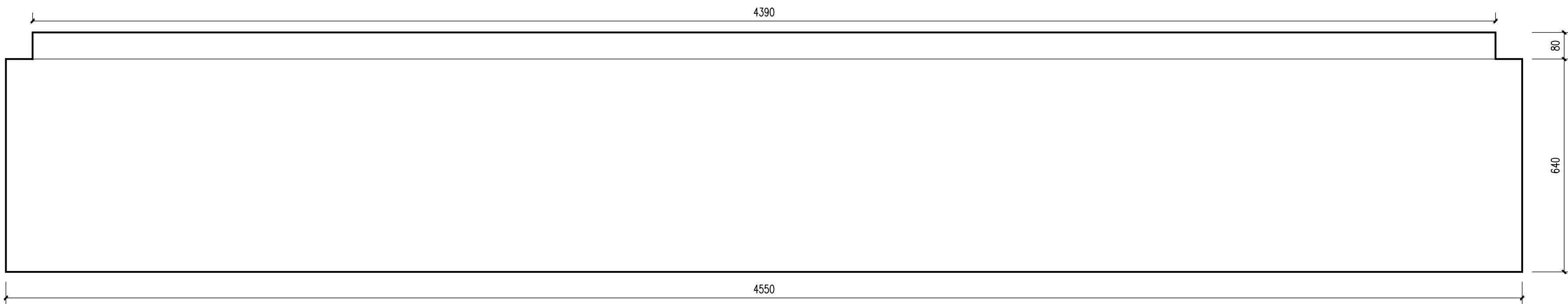
采访台 正面展开图 1:10
