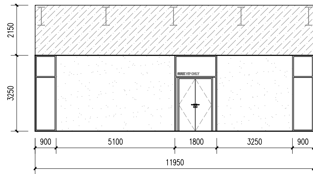
西入口区域 E立面图 1:100
