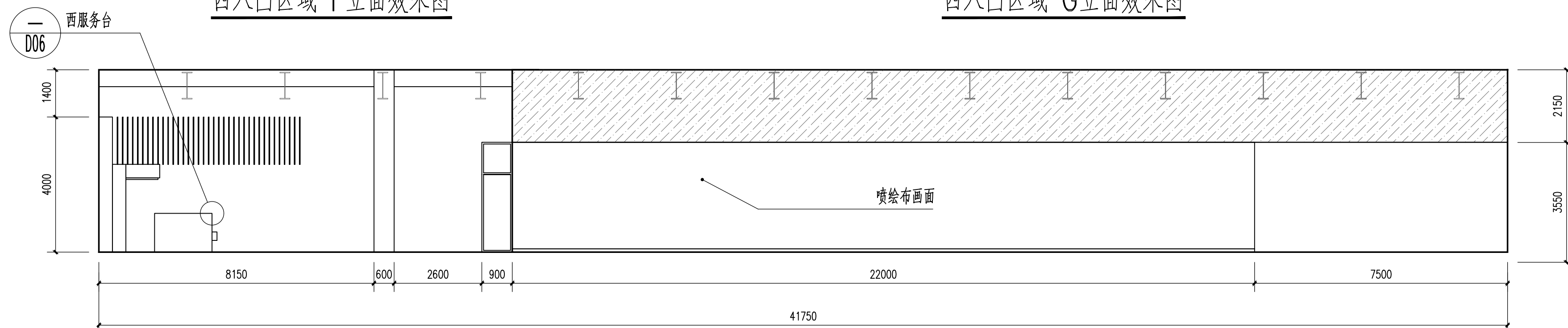
西入口区域 G立面图 1:100
