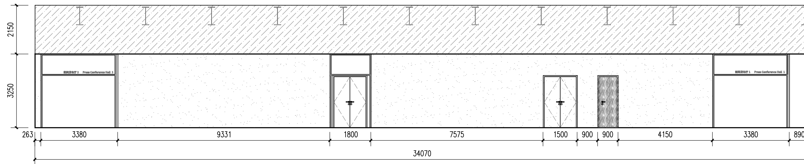
西入口区域 F立面图 1:100
