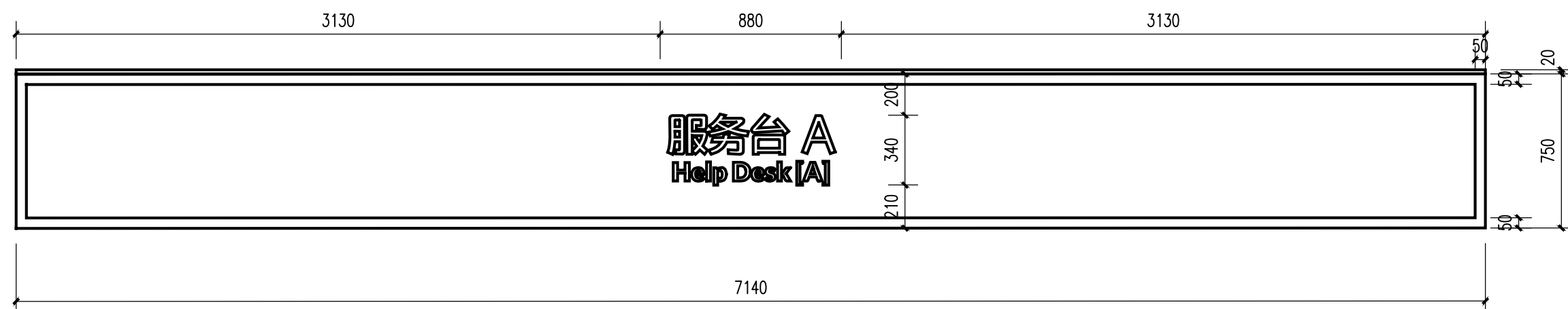
服务台A 前视图 1:25
