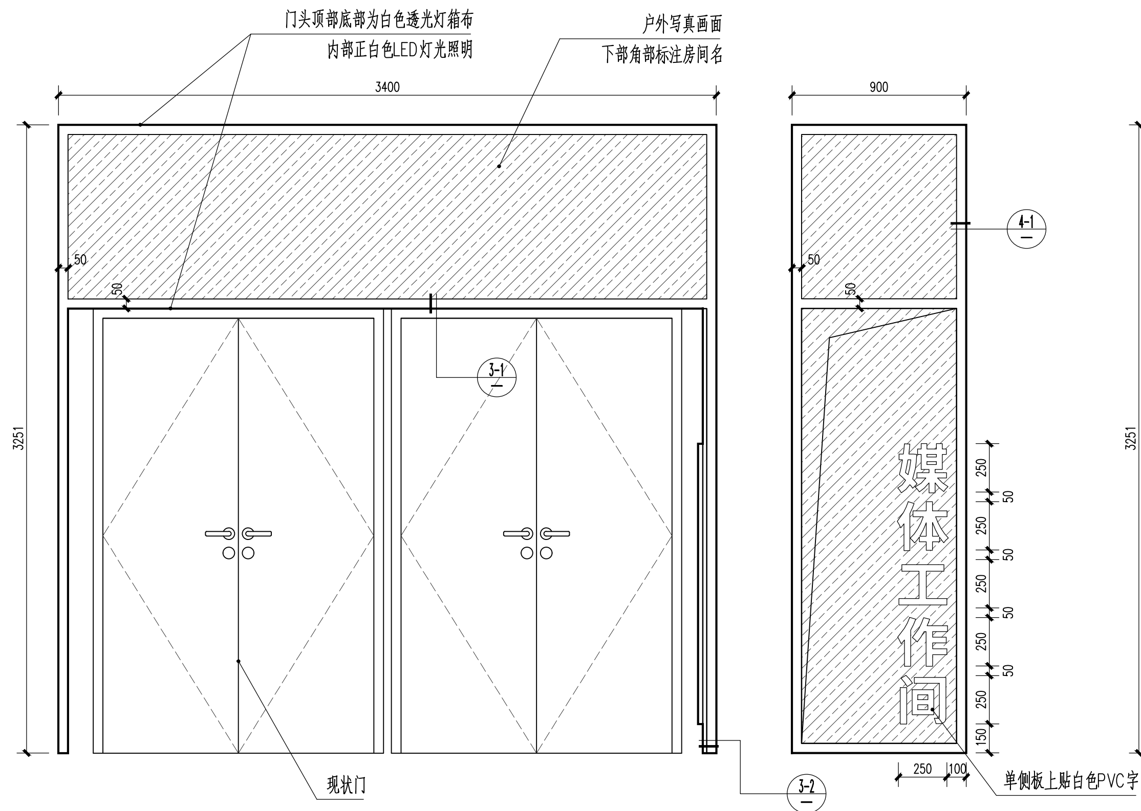
① 门框(大)正、侧立面图 1:20
