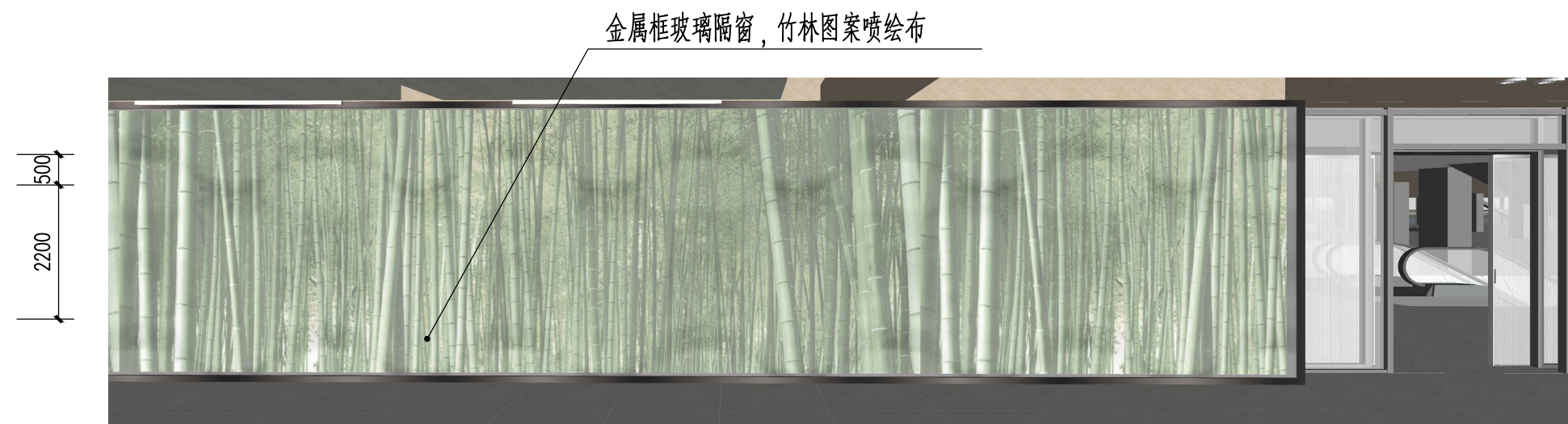
媒体餐厅 F立面图 1:100
