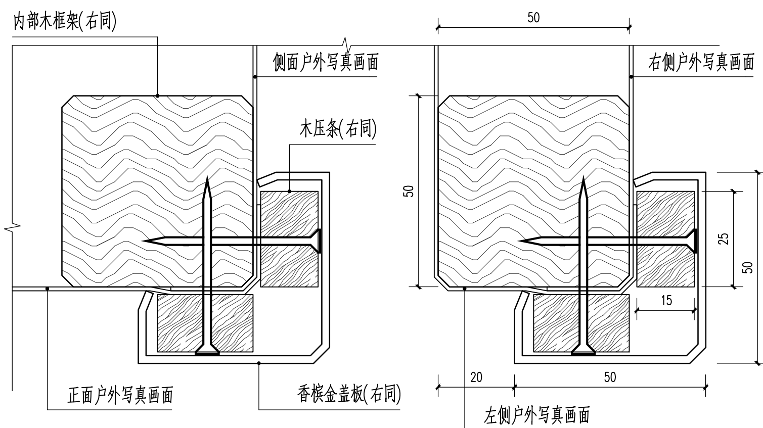
③-1 门框边框(角部)大样图 1:1 ③-2 门框边框(端部)大样图 1:1
