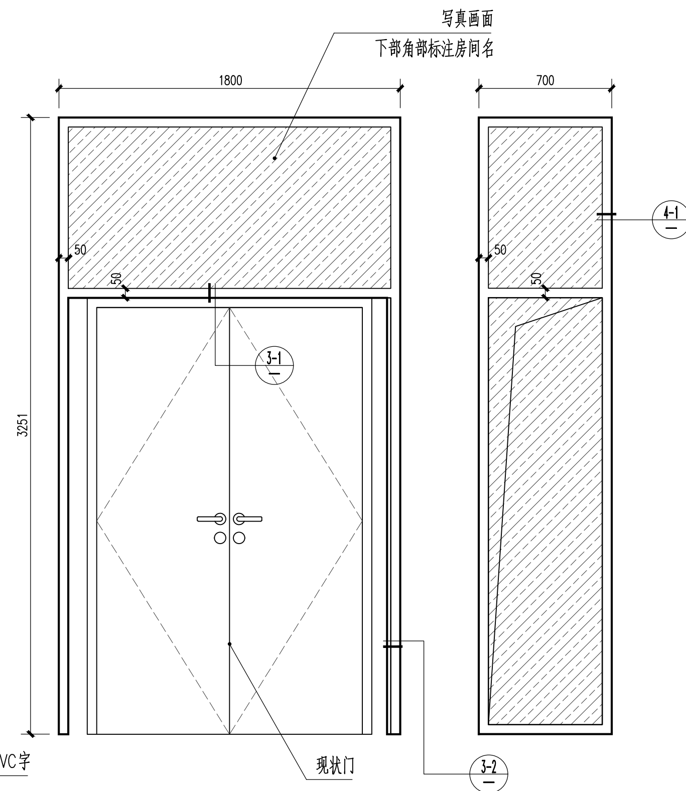
② 门框(小)正、侧立面图 1:20
