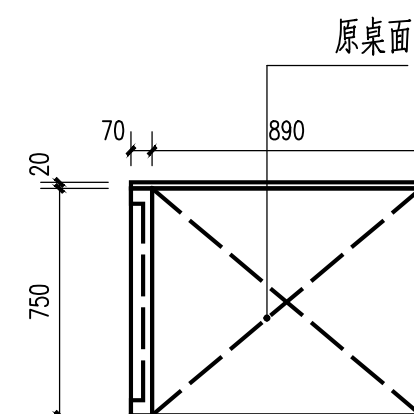
服务台AB 侧视图 1:25
