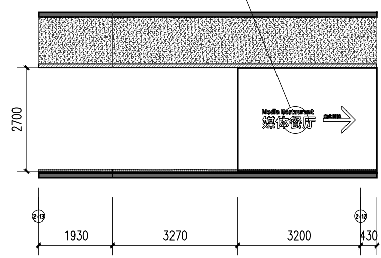
媒体餐厅 B立面图 1:100
