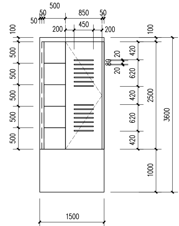
LED屏B 右侧视图 1:50
