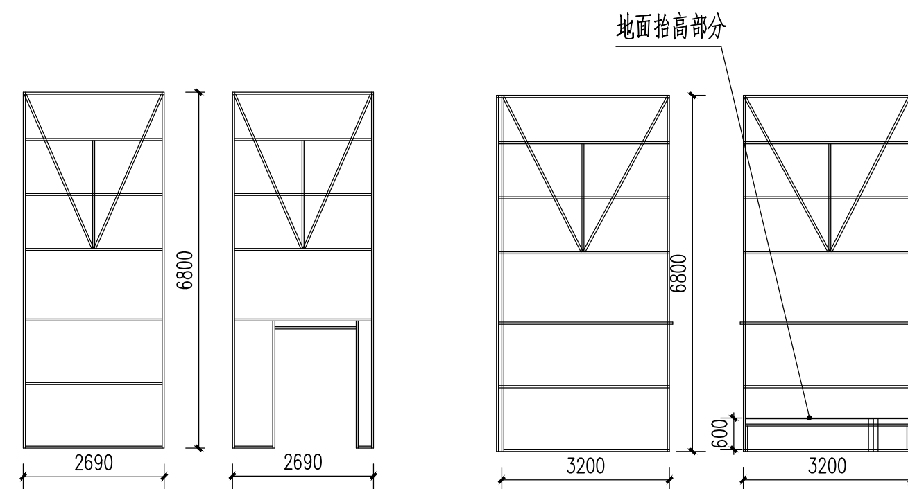
隔墙短边CD立面钢骨架图 1:100
