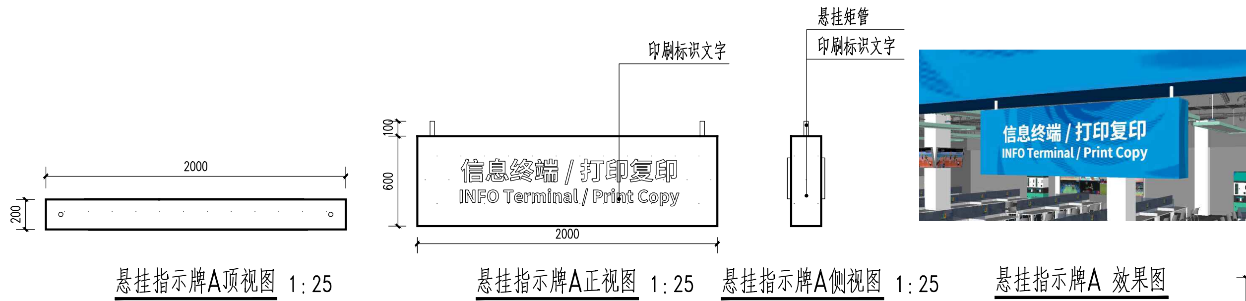
① 悬挂指示牌A大样图 1:25
