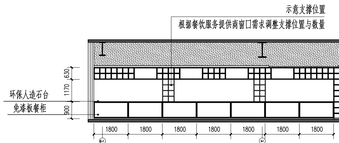
媒体餐厅 E立面图 1:100
