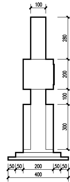
A花箱 侧视图 1:15
