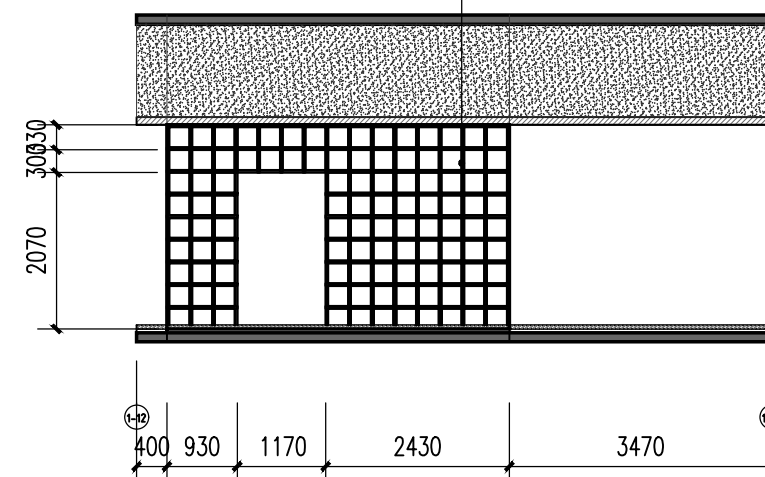
媒体餐厅 C立面图 1:100
