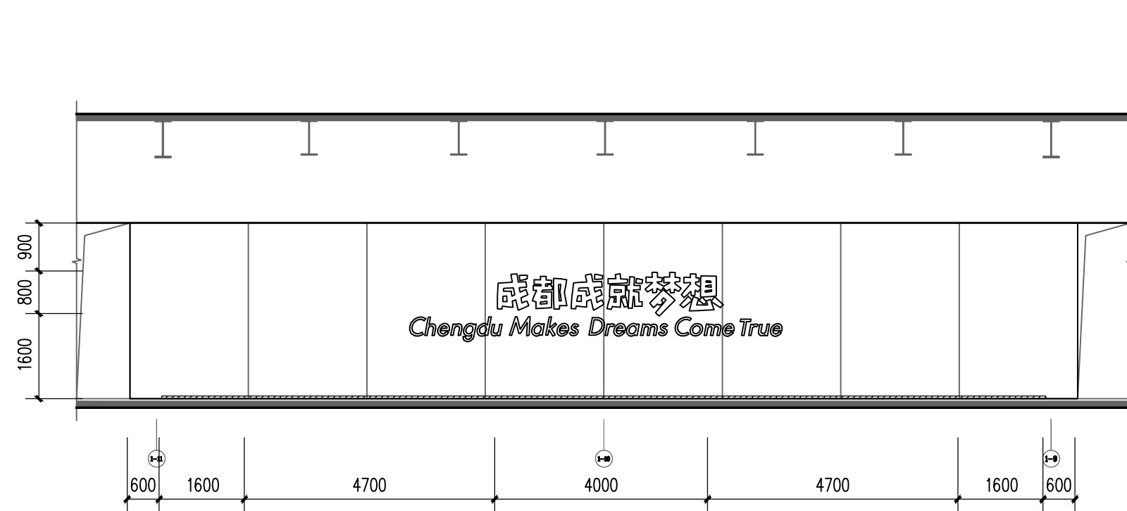
综合服务区 D立面图 1:100
