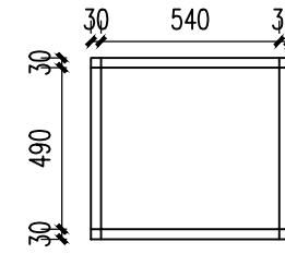
书架标准格子详图 1:25
