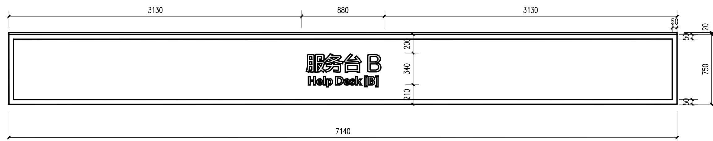
服务台B 前视图 1:25
