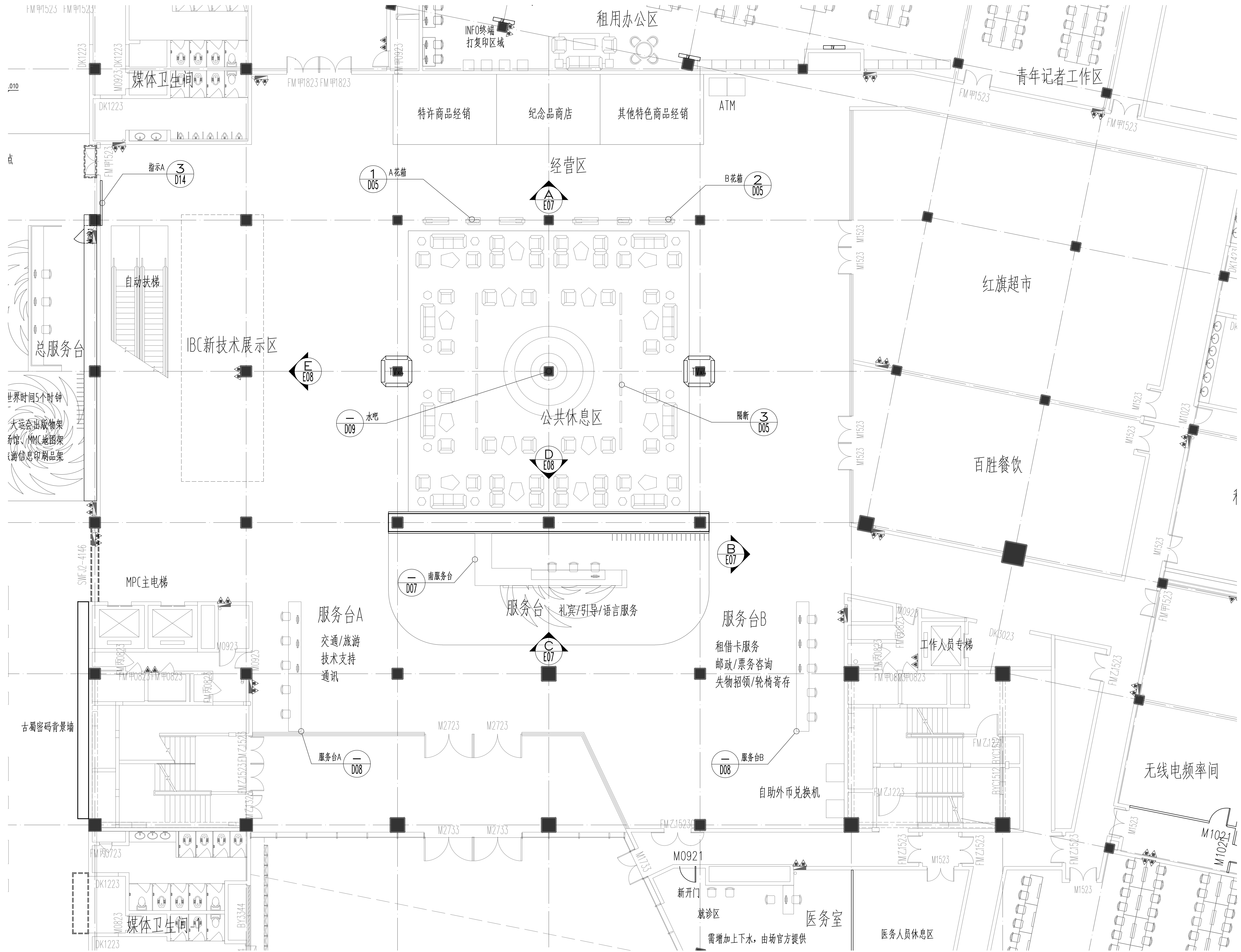
综合服务区放大平面图 1:100
