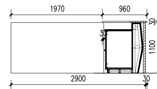
南欢迎台 1-1 剖视图 1:50
