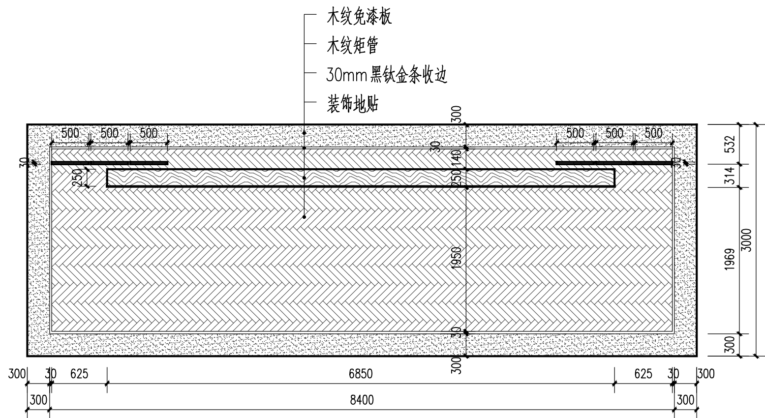
川剧表演舞台顶视图 1:50
