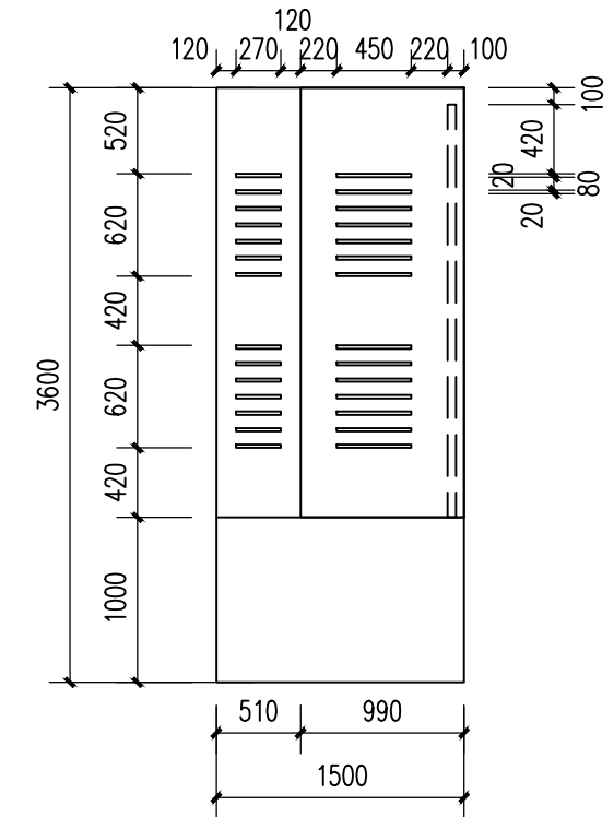
LED屏B 左侧视图 1:50
