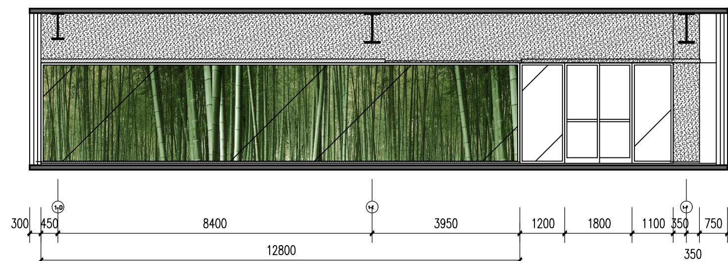
媒体餐厅 G立面图 1:100
