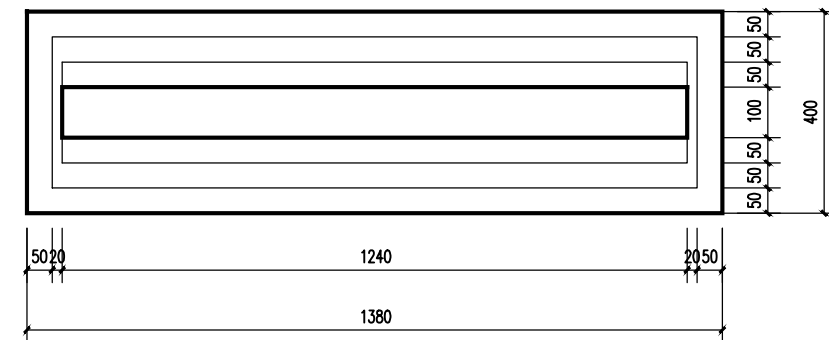
隔断 顶视图 1:15
