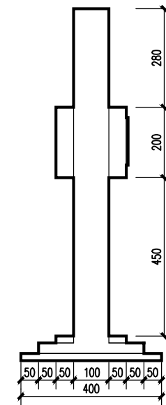
B花箱 侧视图 1:15
