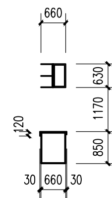
媒体餐厅取餐台剖面图 1:100
