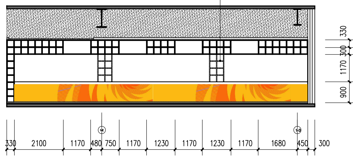
媒体餐厅 D立面图 1:100
