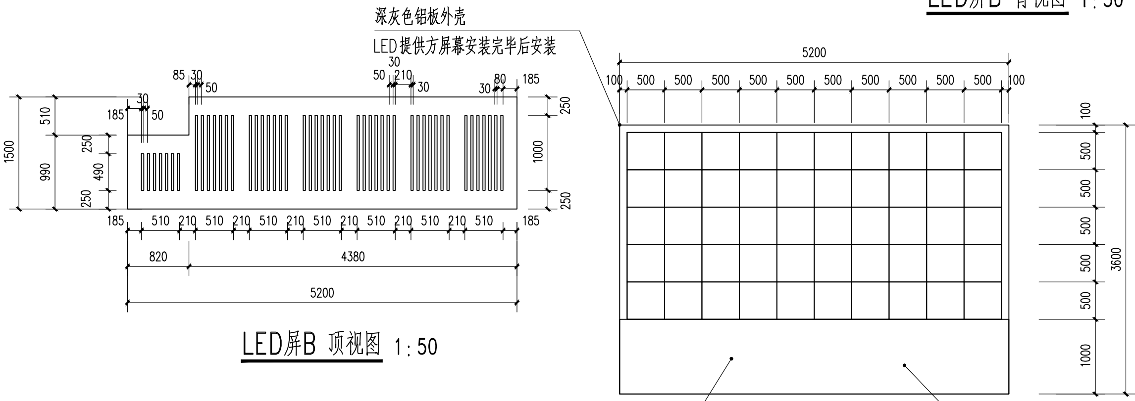
LED屏B 背视图 1:50
