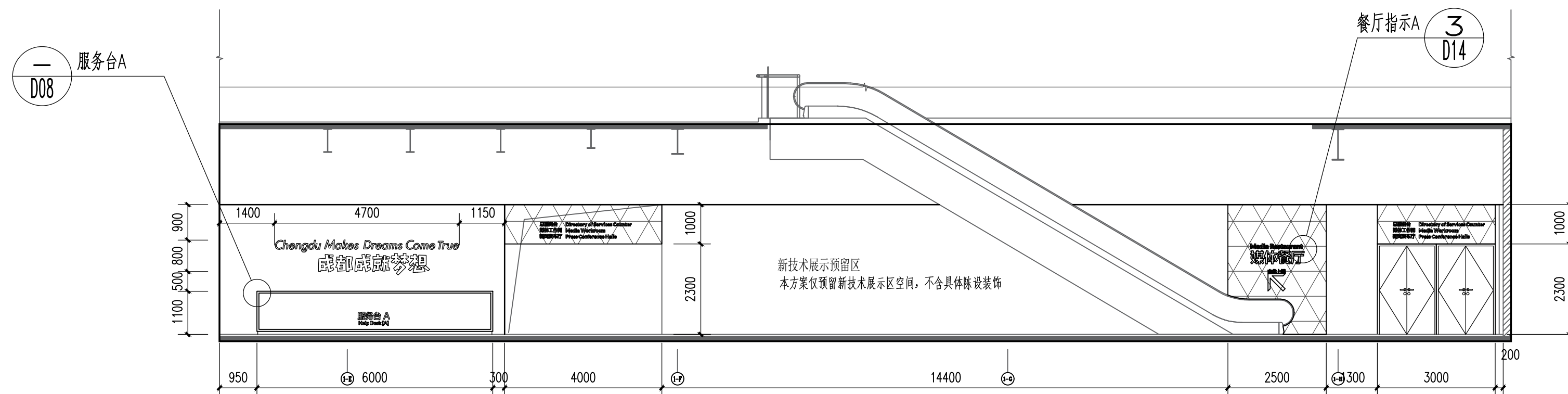
综合服务区 E立面图 1:100
