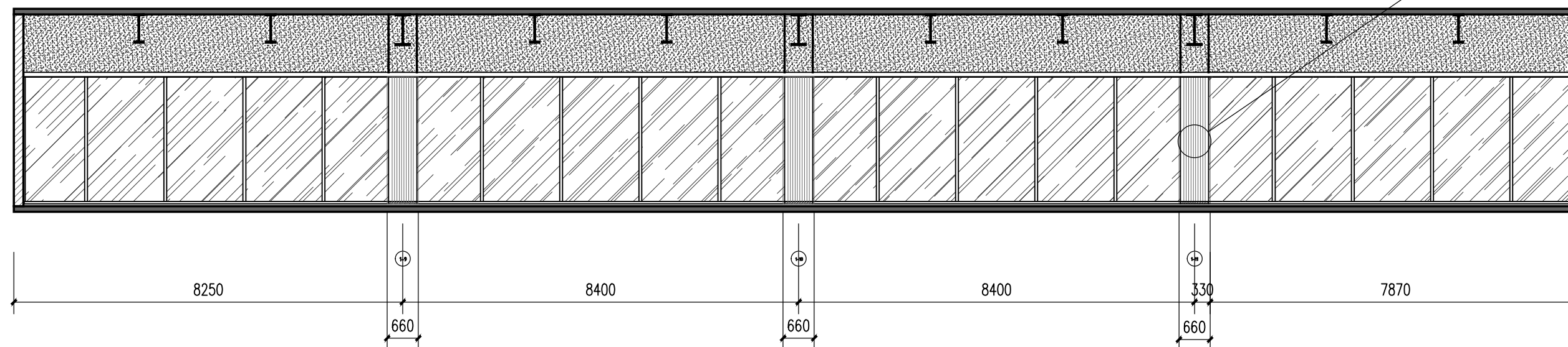
媒体餐厅 A立面图 1:100
