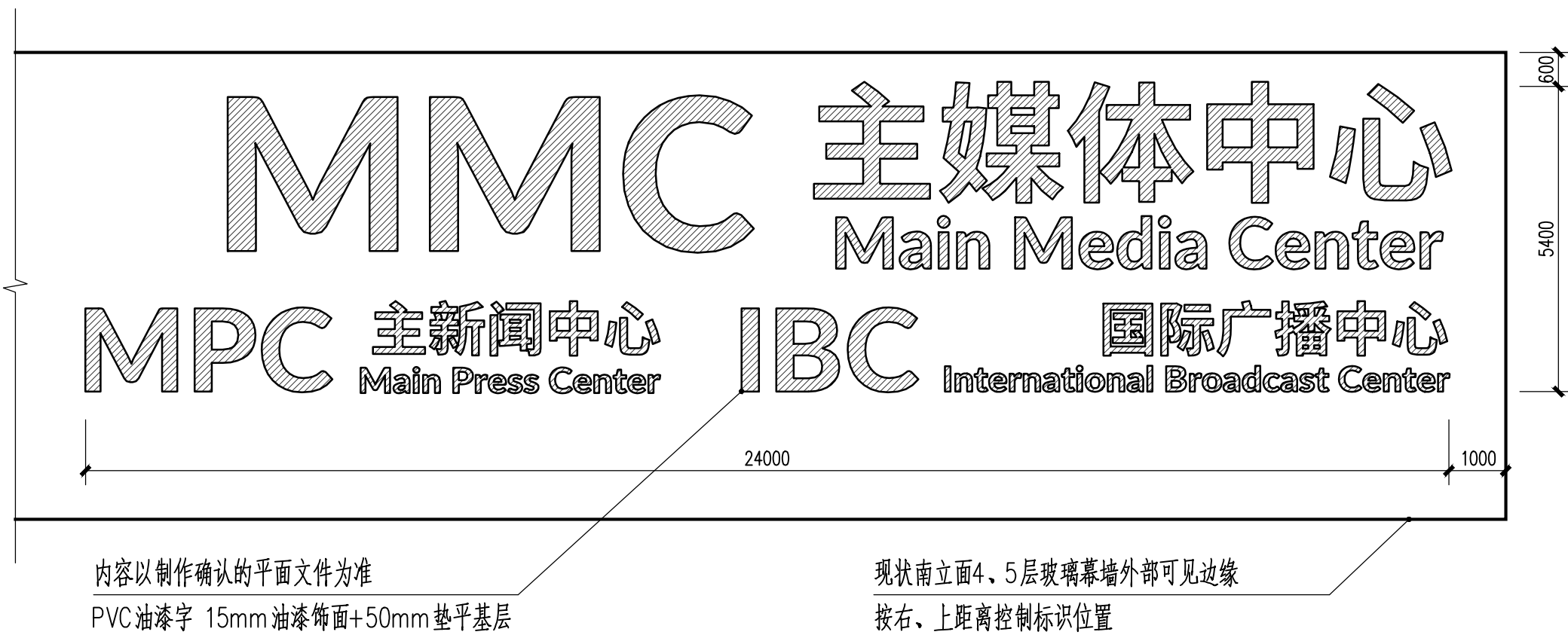
③ 南立面标识立面图 1:100
