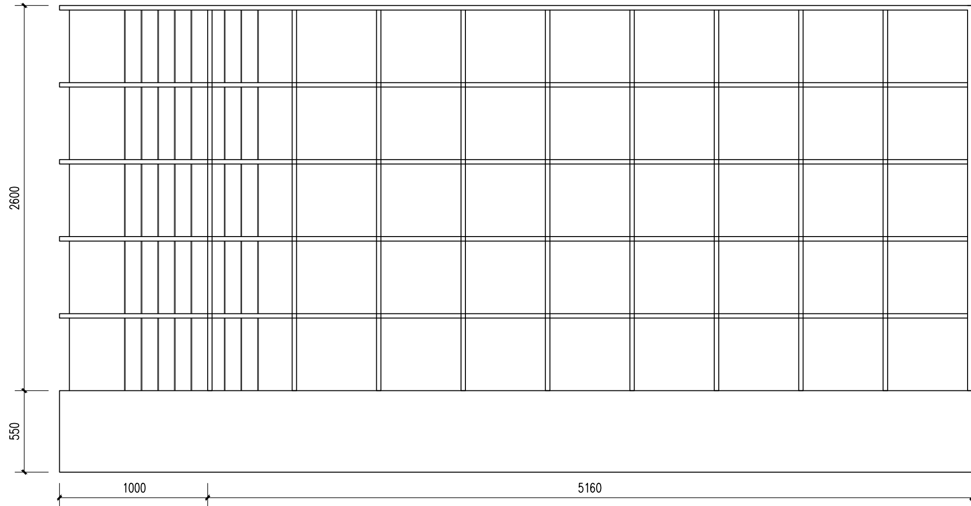
书架 B 立面视图 1:25
