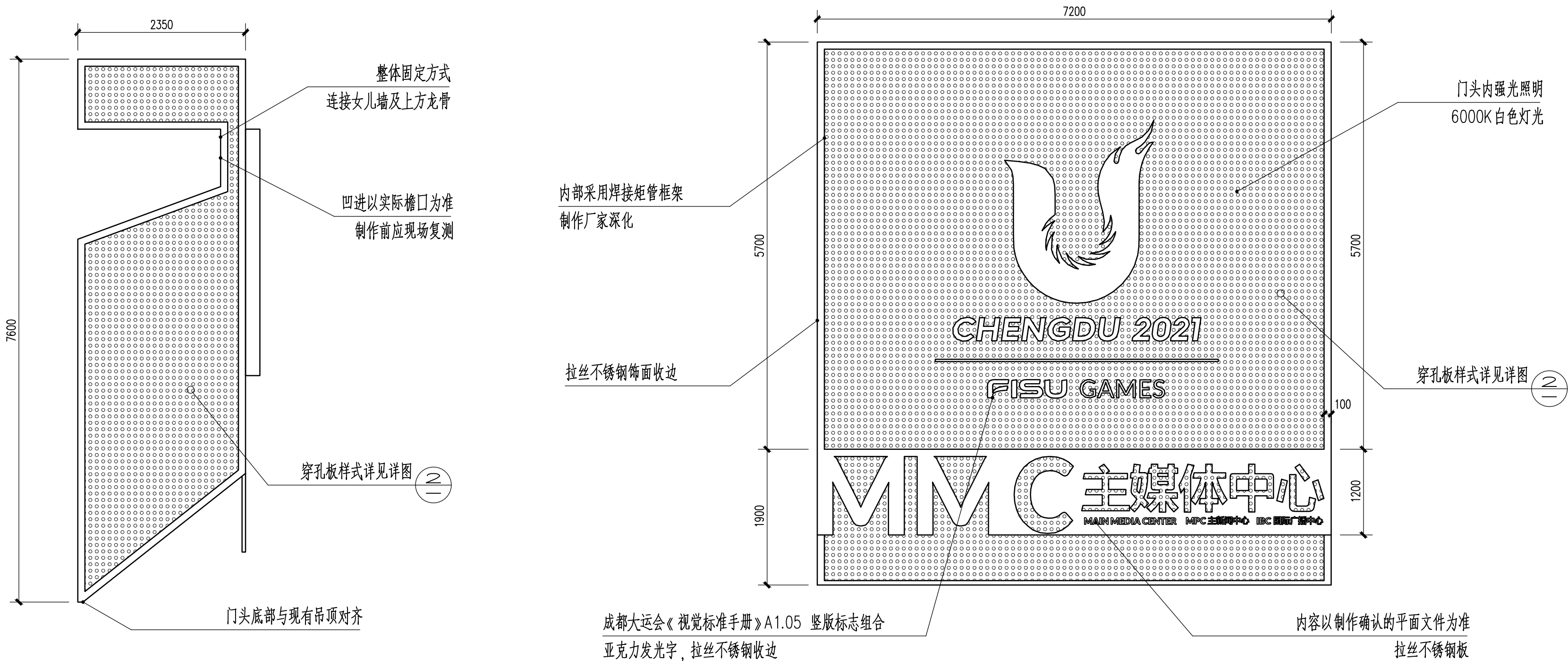
西入口门头侧视图 1:100
