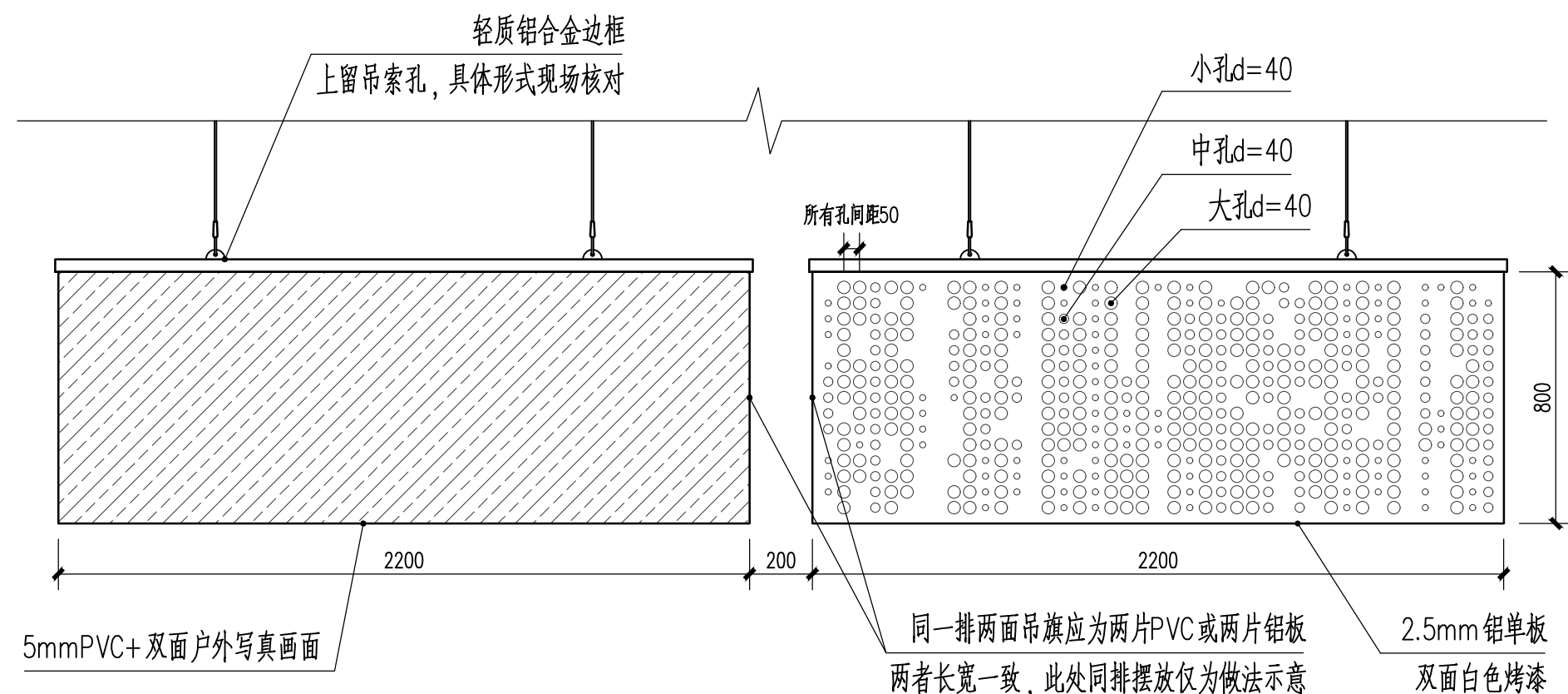
④ 吊旗大样图 1:20
