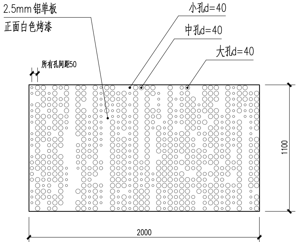
② 西入口门头穿孔板样式图 1:20
