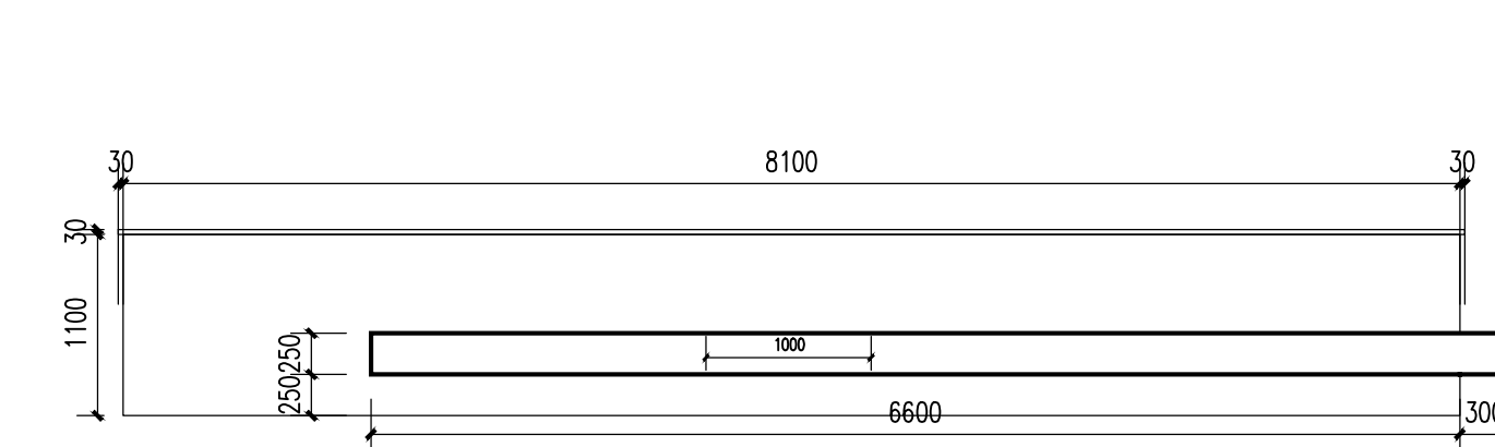
南欢迎台 前视图 1:50
