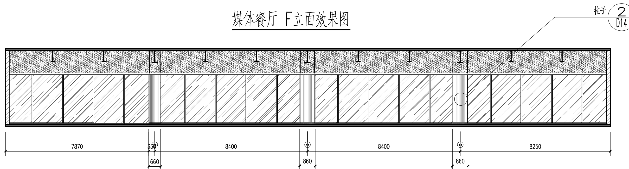
媒体餐厅 F立面图 1:100
